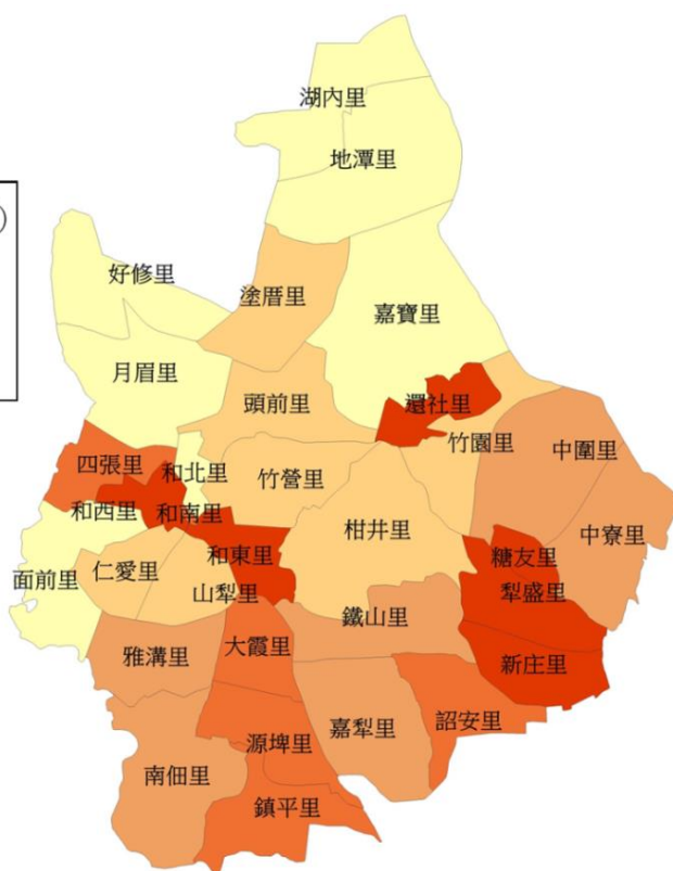
圖 1-3-6 土壤液化分布圖
