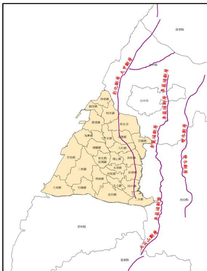
圖 1-3-4 彰化縣附近斷層分布圖
