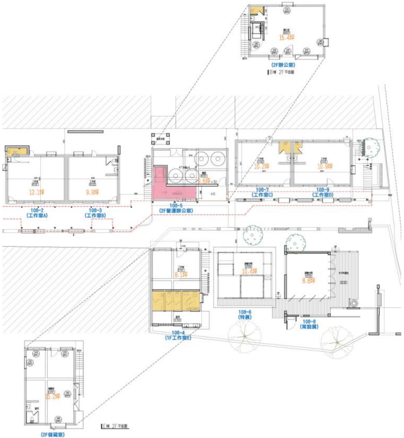
圖一、和興青創基地空間示意圖
